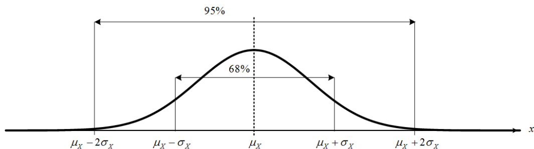
圖 3: 常態機率分布圖
